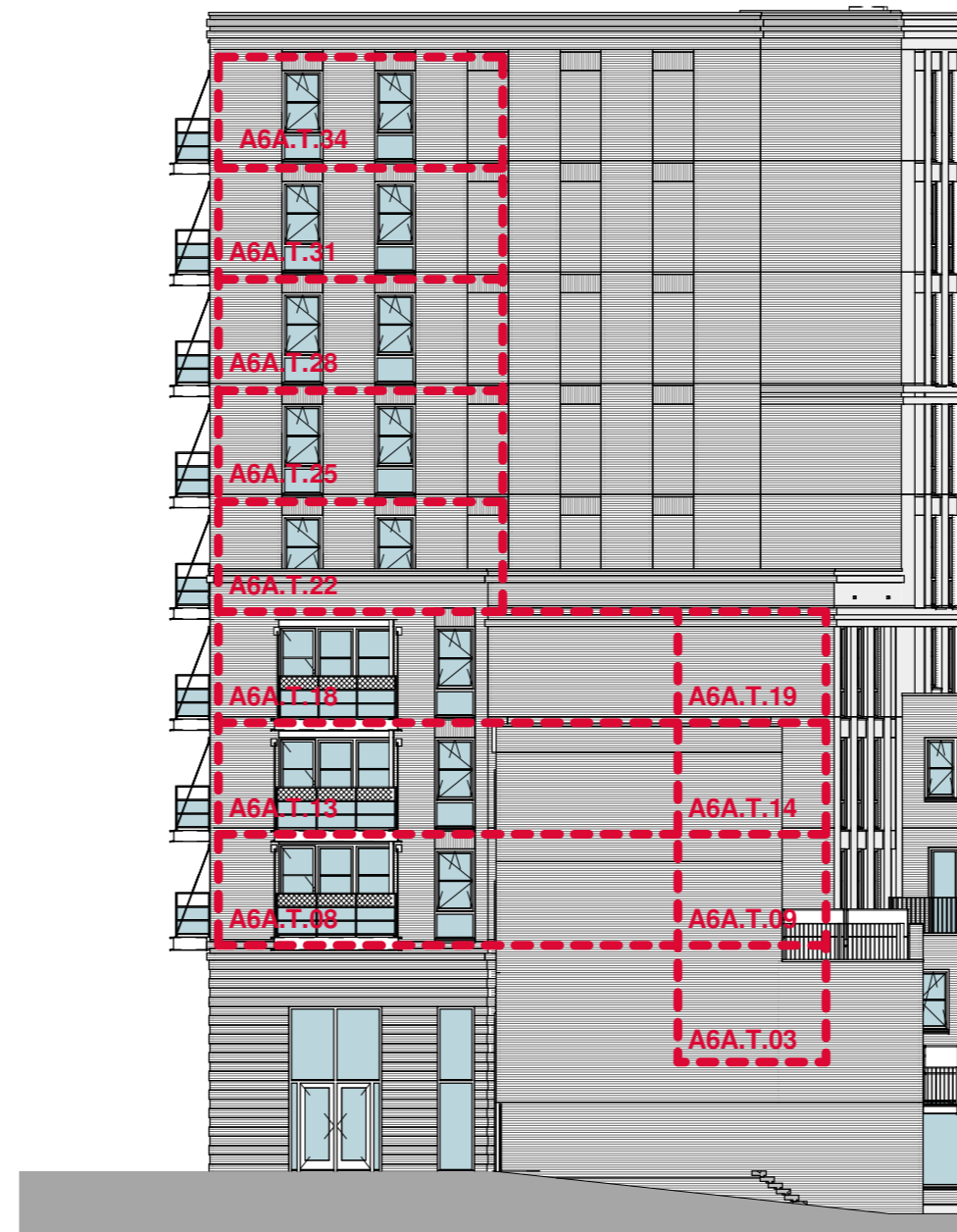
Blok A6-A Oostgevel
