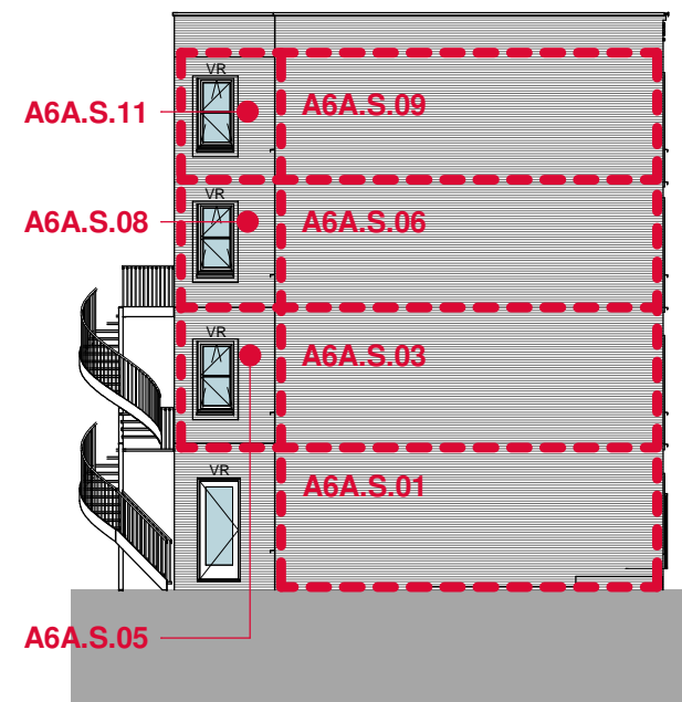
A6-A Oostgevel
